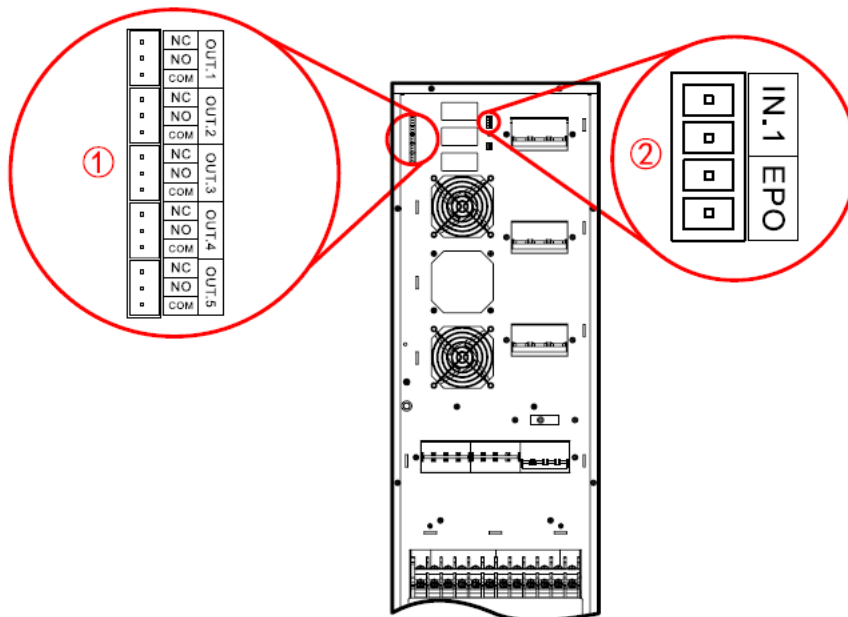
Рис 2-15 Расположение сухих контактов для ИБП 30/40/
