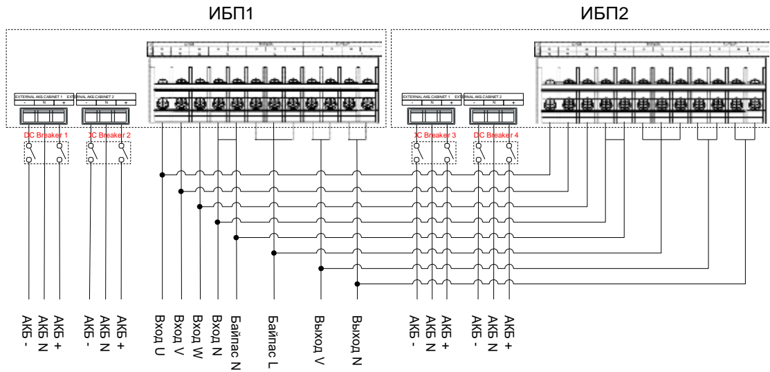
Рис. 3-30 30/40 диаграмма подключения для 31 режима параллельной системы
