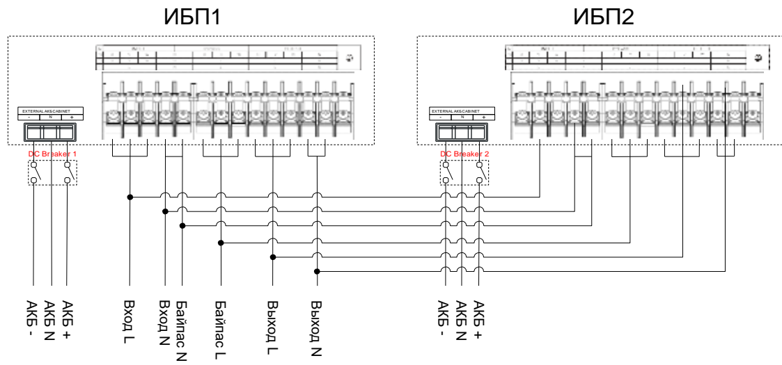
Рис. 3-28 10/15/20 диаграмма подключения для 11 режима параллельной системы
