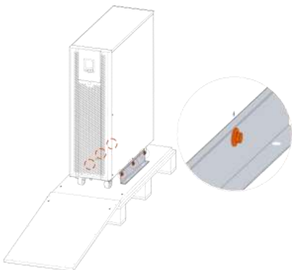
Рис. 3-5 Расположение болтов
