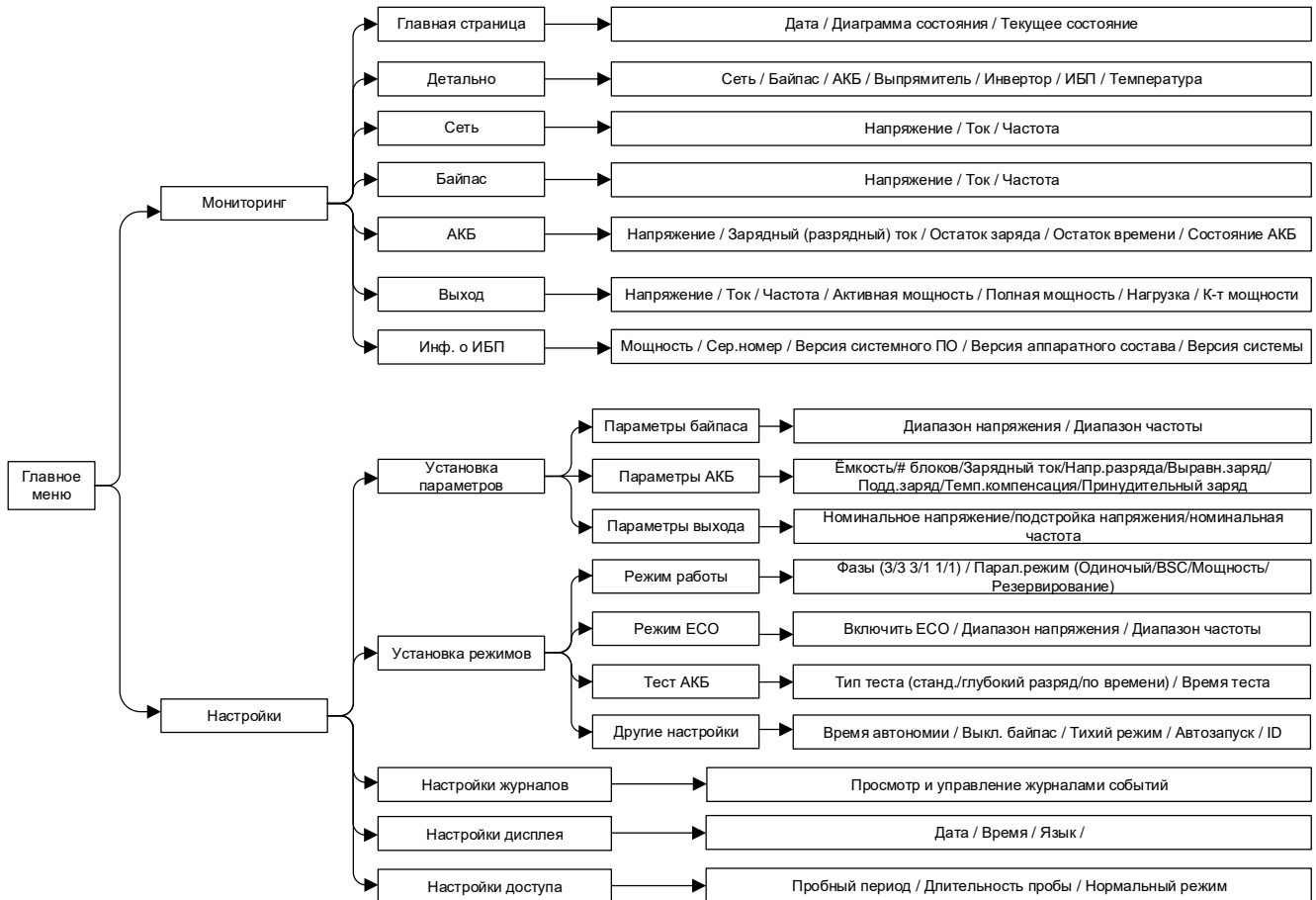
Рис 4-1 Структура меню ИБП с сенсорным экраном
