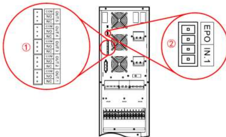
Рис 2-14 Расположение сухих контактов для ИБП 10/15/20
