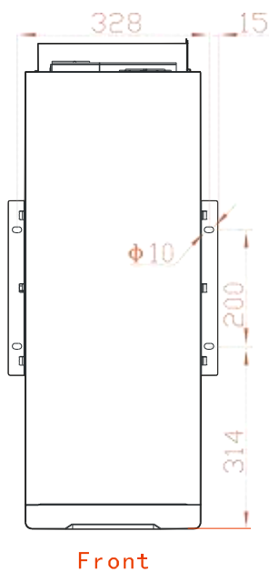
Рис. 3-9 30/30С/40/40С отверстия для монтажа в раме ИБП (вид сверху)
