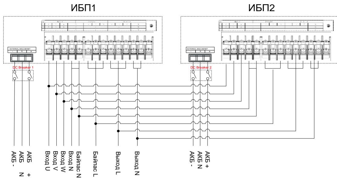
Рис. 3-27 10/15/20 диаграмма подключения для 31 режима параллельной системы
