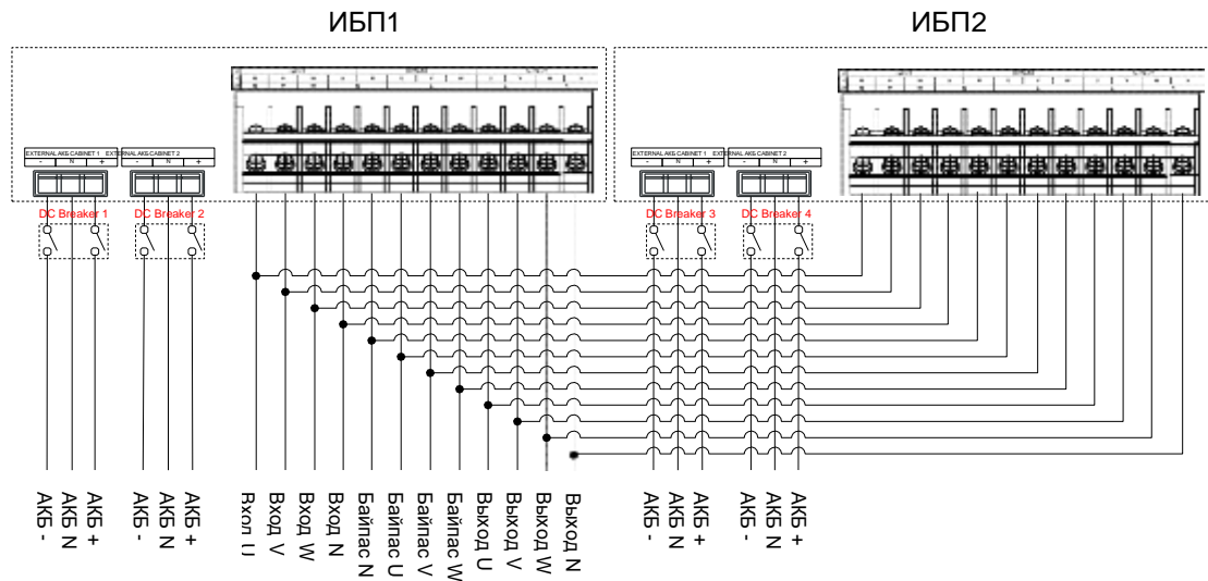
Рис. 3-29 30/40 диаграмма подключения для 33 режима параллельной системы
