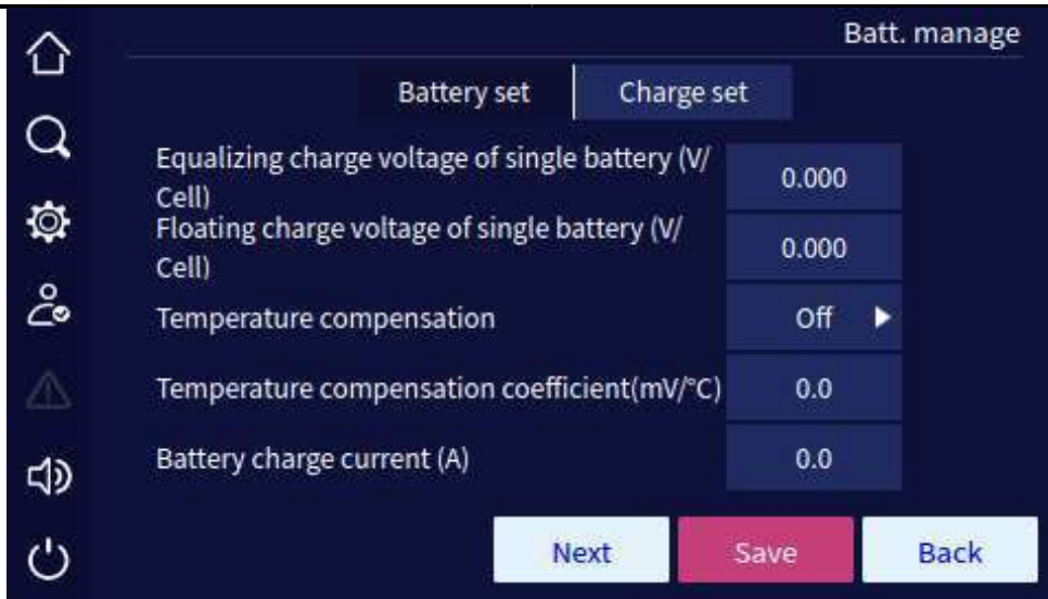
Рис 4.32 Настройка заряда АКБ 1
