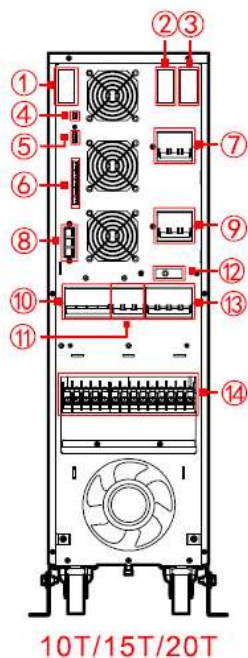
Рис 2-6 Вид задней панели моделей 10/10С/15/15С/20/20С
