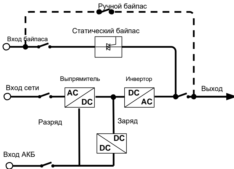
Рис. 2-9 Функциональная диаграмма
