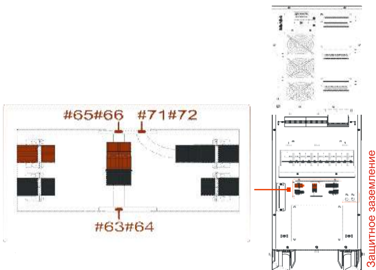
Рис. 3-20 Подключение установочной перемычки по умолчанию
