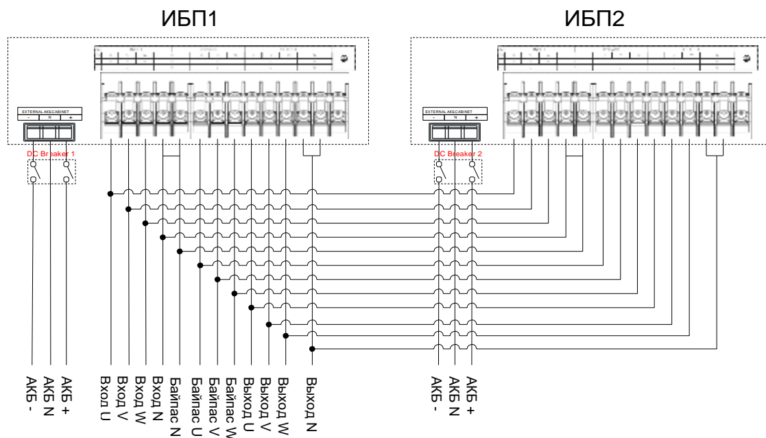
Рис. 3-26 10/15/20 диаграмма подключения 33 режим для параллельной системы
