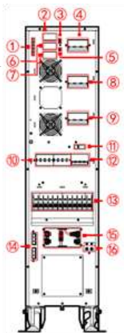
Рис 2-7 Вид задней панели моделей АБ-КР33 30/ АБ-КР33 30С
