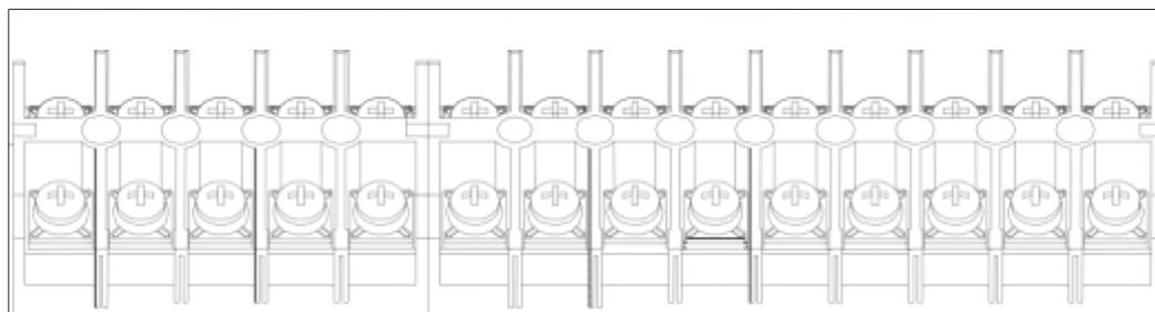
Рис. 3-13 Маркировка кабельных клемм
