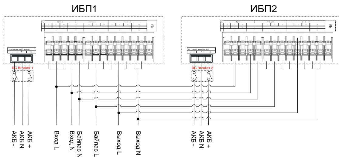
Рис. 3-28 АБ-КР33 10/ АБ-КР33 10С/ АБ-КР33 15/ АБ-КР33 15С/ АБ-КР33 20/ АБ-КР33 20С диаграмма подключения для 11 режима параллельной системы
