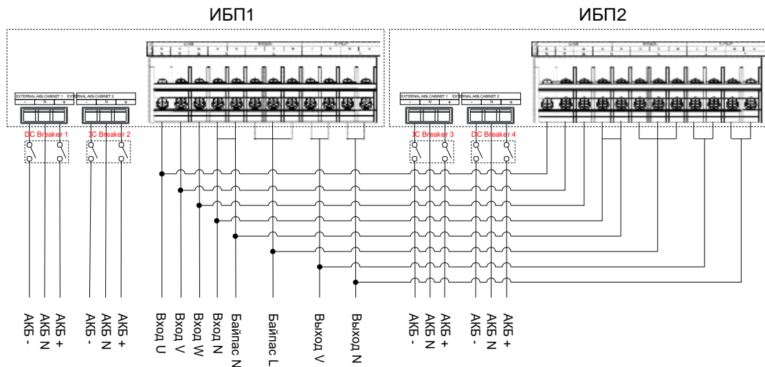
Рис. 3-30 АБ-КР33 30/ АБ-КР33 30С/ АБ-КР33 40/ АБ-КР33 40С диаграмма подключения для 31 режима параллельной системы
