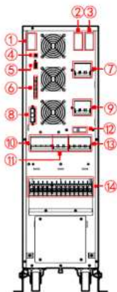
Рис 2-6 Вид задней панели моделей АБ-КР33 10/ АБ-КР33 10С/ АБ-КР33 15/ АБ-КР33 15С/ АБ-КР33 20/ АБ-КР33 20С
