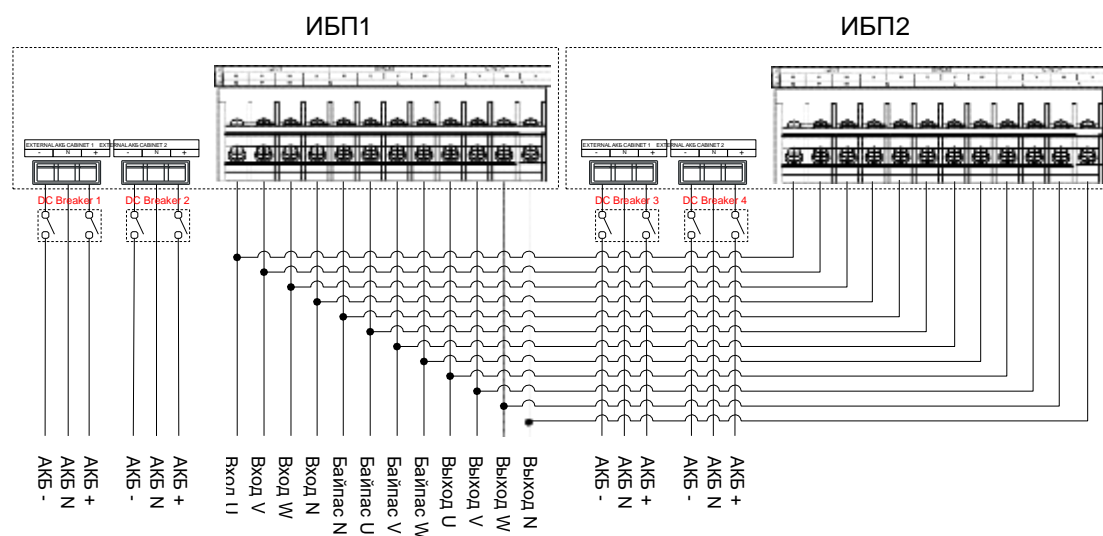
Рис. 3-29 АБ-КР33 30/ АБ-КР33 30С/ АБ-КР33 40/ АБ-КР33 40С диаграмма подключения для 33 режима параллельной системы
