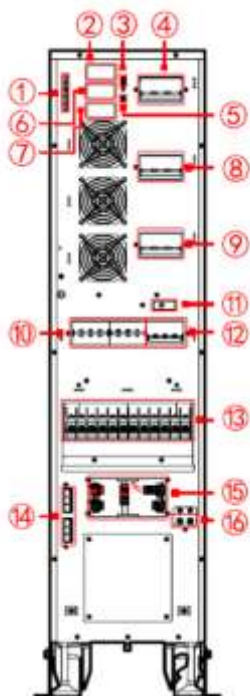
Рис 2-8 Вид задней панели моделей АБ-КР33 40/ АБ-КР33 40С
