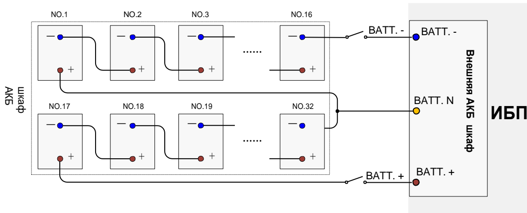
Рис. 3-24 Диаграмма подключения одного батарейного шкафа
