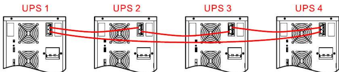
Рис. 3-32 Диаграмма подключения информационных кабелей параллельной системы из четырёх ИБП
