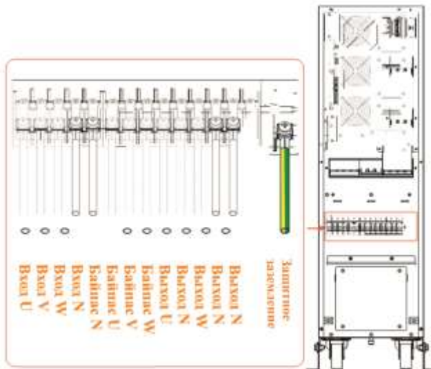
Рис. 3-14 Диаграмма подключения для 33 режима
