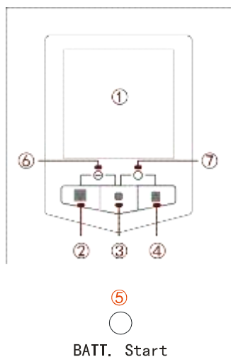
Рис. 2-4 Панель управления с ЖК дисплеем
