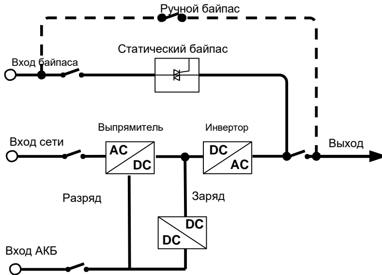
Рис. 2-9 Функциональная диаграмма
