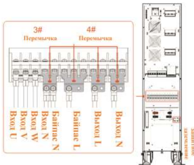
Рис. 3-23 Медные перемычки и диаграмма подключения для 31 режима
