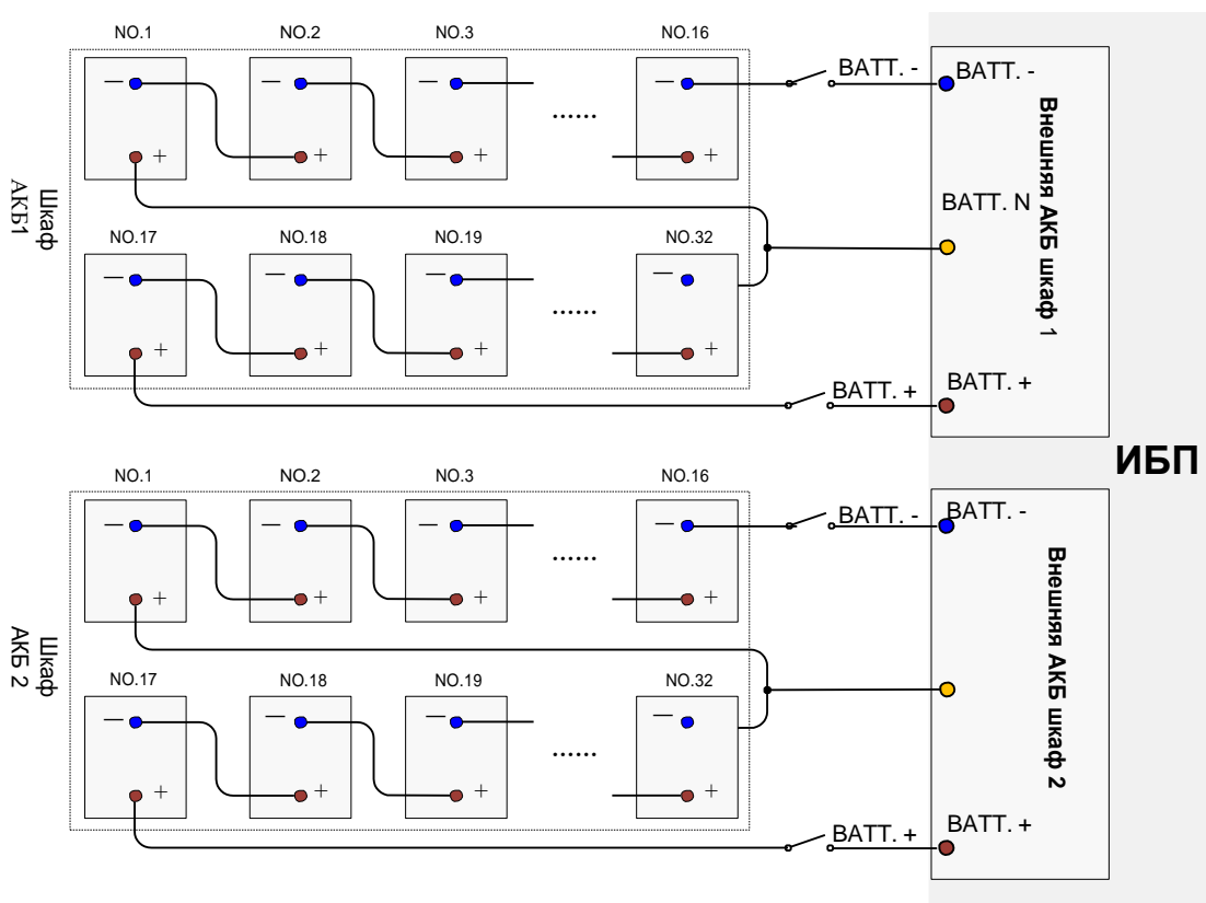
Рис. 3-25 Диаграмма подключения двух батарейных шкафов
