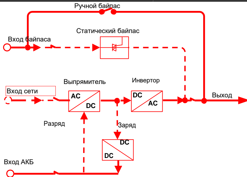
Рис 2-13 Режим ручного байпаса (жирная линия показывает поток энергии)
