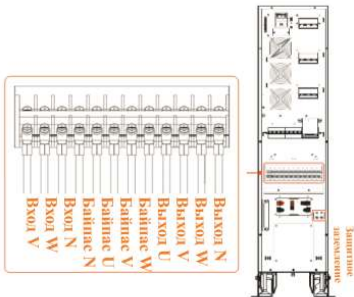
Рис. 3-21 Диаграмма подключения для 33 режима
