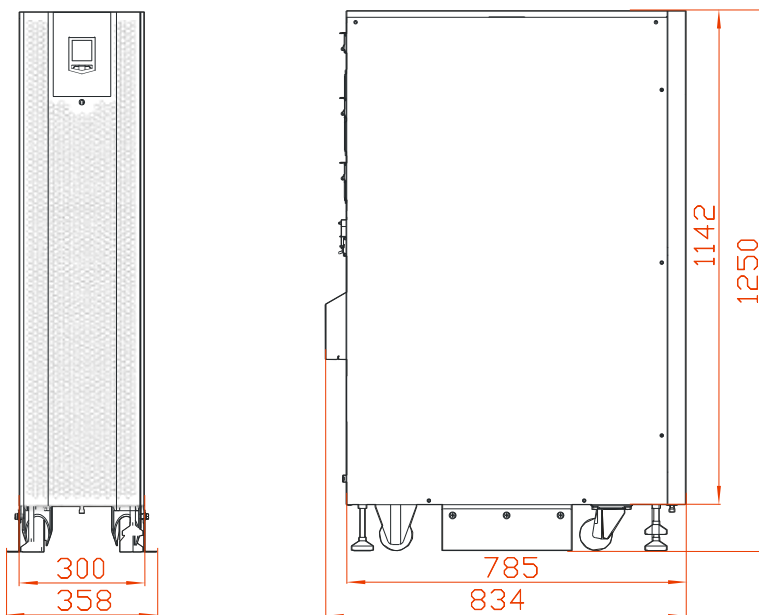
Рис. 3-7 Внешние размеры ИБП АБ-КР33 30/ АБ-КР33 30С/ АБ-КР33 40/ АБ-КР33 40С
