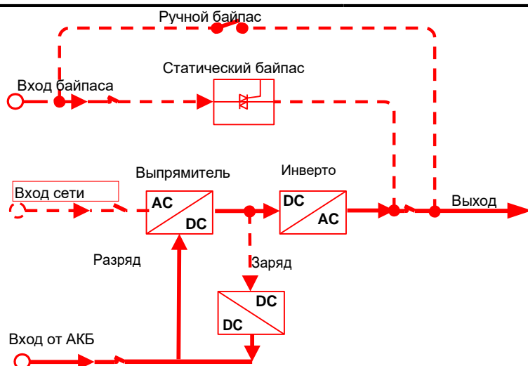
Рис 2-11 Режим работы от АКБ (жирная линия показывает поток энергии)
