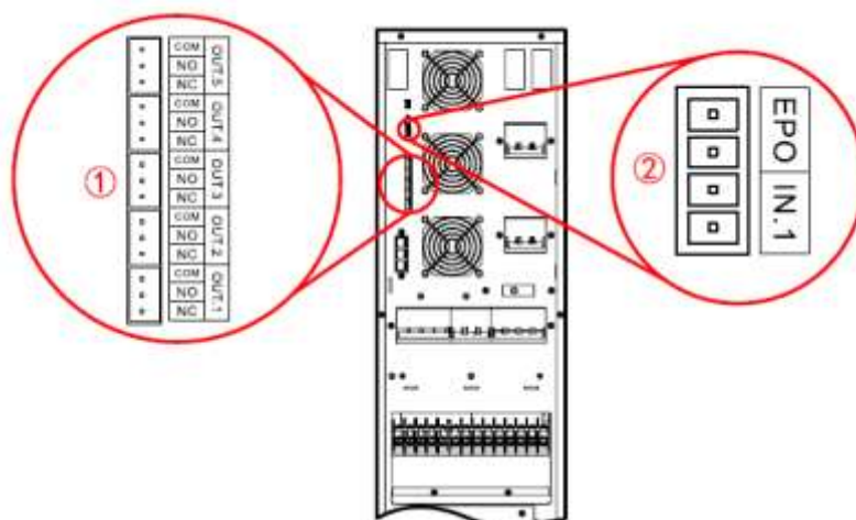
Рис 2-14 Расположение сухих контактов для ИБП АБ-КР33 10/ АБ-КР33 10С/ АБ-КР33 15/ АБ-КР33 15С/ АБ-КР33 20/ АБ-КР33 20С
