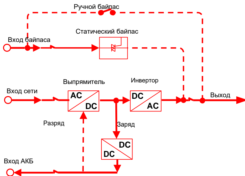
Рис 2-10 Нормальный режим работы от сети (жирная линия показывает поток энергии)
