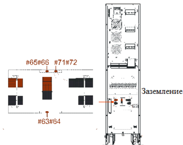
Рис. 3-20 Подключение установочной перемычки по умолчанию
