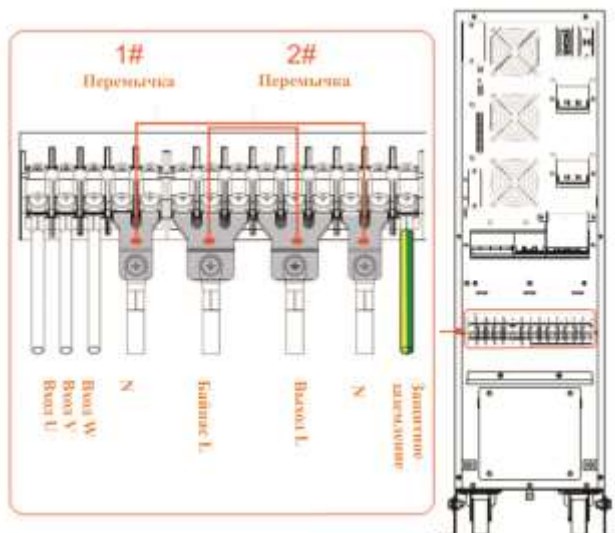
Рис. 3-15 Установка перемычек и подключение кабелей для 31 режима
