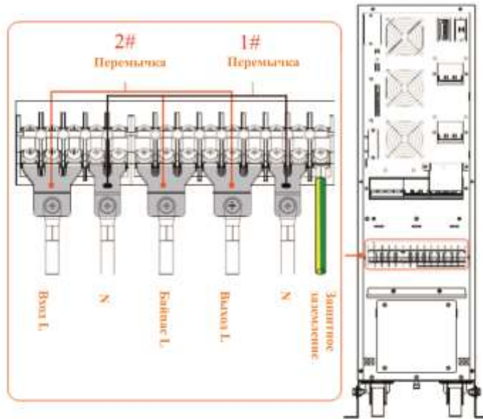
Рис. 3-16 Установка перемычек и подключение кабелей для 11 режима
