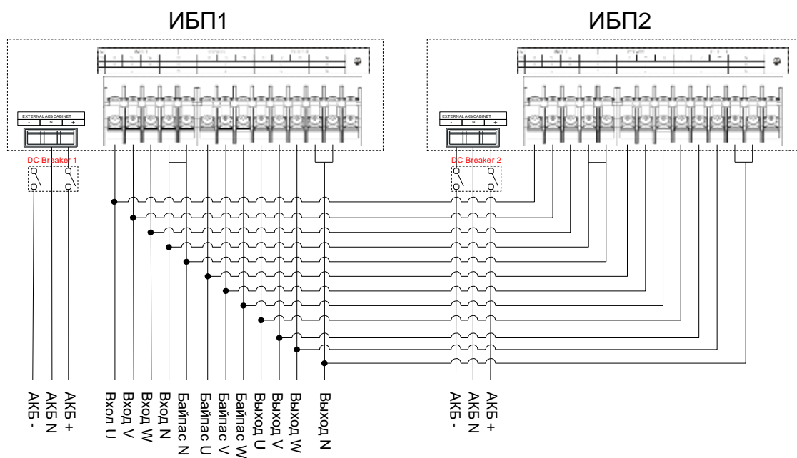
Рис. 3-26 АБ-КР33 10/ АБ-КР33 10С/ АБ-КР33 15/ АБ-КР33 15С/ АБ-КР33 20/ АБ-КР33 20С диаграмма подключения 33 режим для параллельной системы
