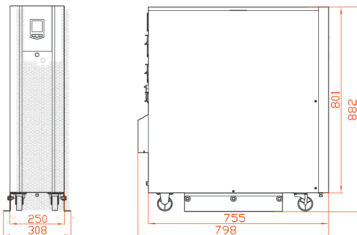
Рис. 3-6 Внешние размеры ИБП АБ-КР33 10/ АБ-КР33 10С/ АБ-КР33 15/ АБ-КР33 15С/ АБ-КР33 20/ АБ-КР33 20С
