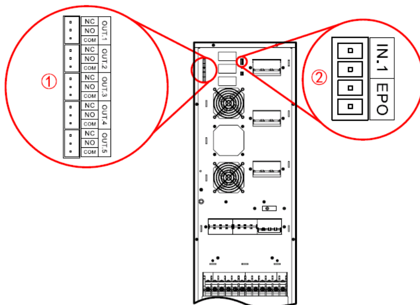
Рис 2-15 Расположение сухих контактов для ИБП АБ-КР33 30/ АБ-КР33 30С/ АБ-КР33 40/ АБ-КР33 40С
