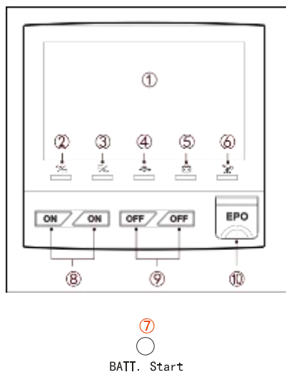
Рис 2-5 Панель управления с сенсорным дисплеем
