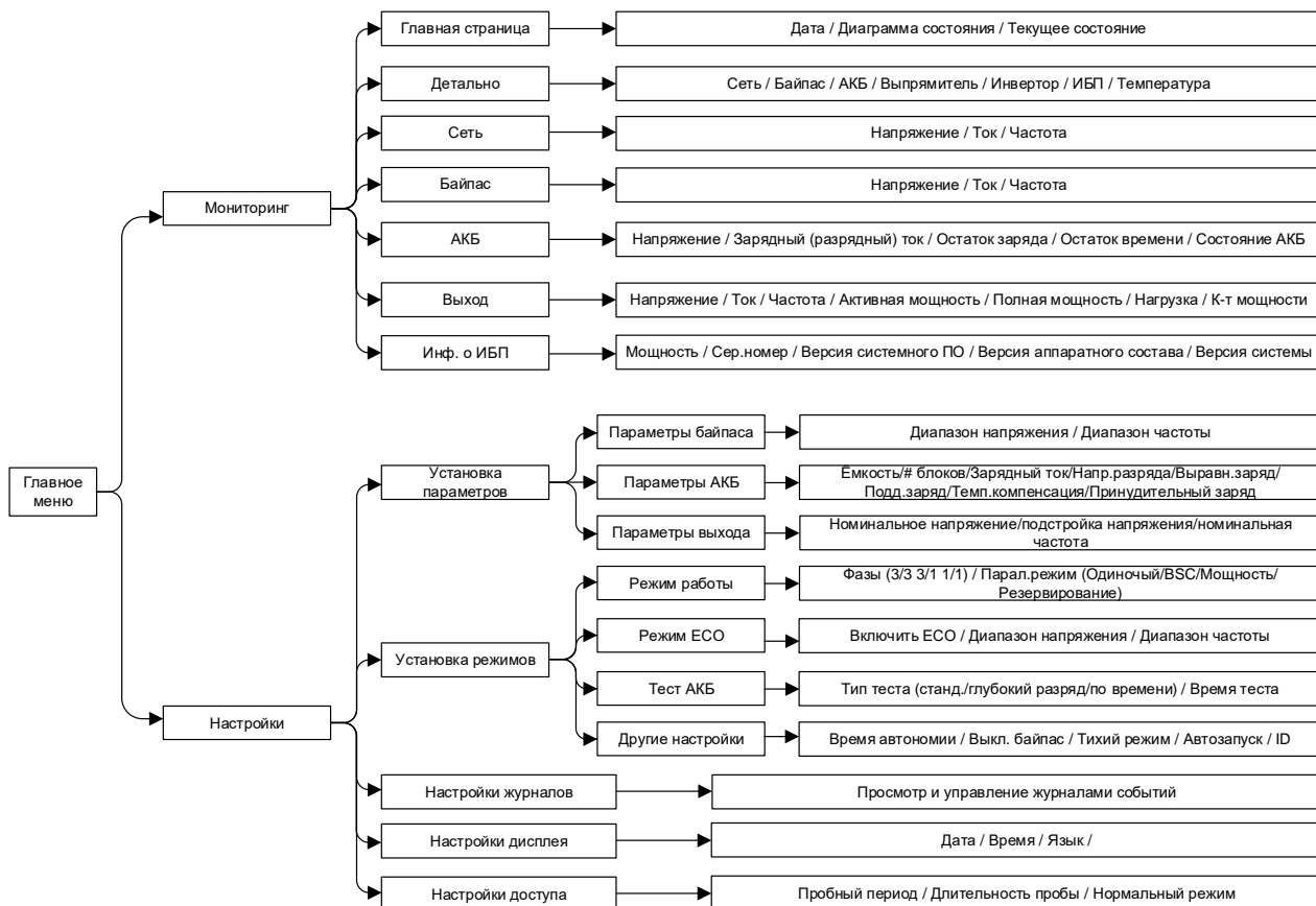
Рис 4-1 Структура меню ИБП с сенсорным экраном
