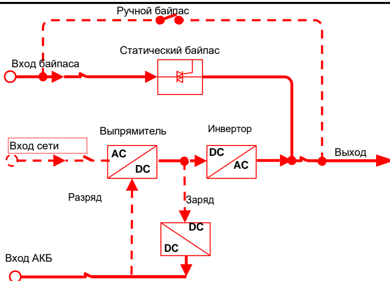
Рис 2-12 Режим работы через байпас ((жирная линия показывает поток энергии))
