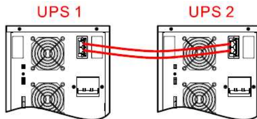
Рис. 3-31 Диаграмма подключения информационных кабелей параллельной системы из двух ИБП
