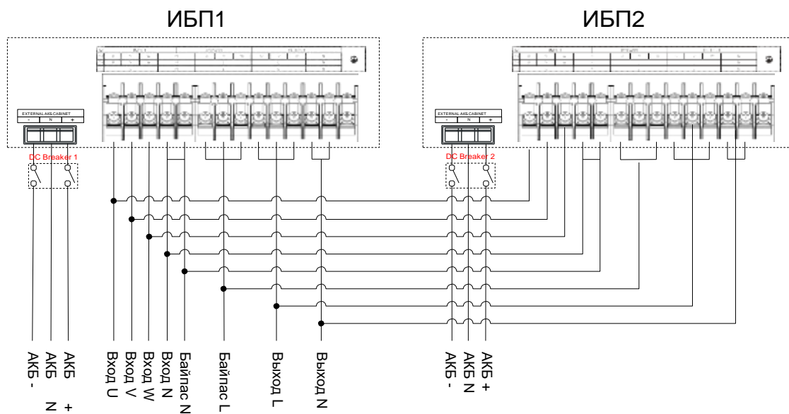
Рис. 3-27 АБ-КР33 10/ АБ-КР33 10С/ АБ-КР33 15/ АБ-КР33 15С/ АБ-КР33 20/ АБ-КР33 20С диаграмма подключения для 31 режима параллельной системы
