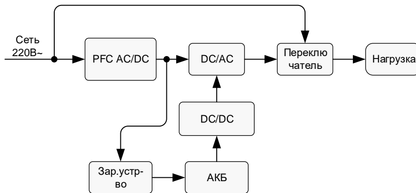
Рис 2.6 Принципиальная рабочая схема для АБ-КР Л 11/6000+, АБ-КР 11/10000+
