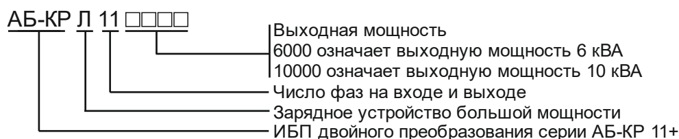
Рис 2.1 Обозначение ИБП
