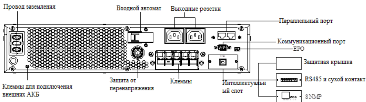
Рис 2.5 Задняя панель для АБ-КР Л 11/6000+, АБ-КР 11/10000+
