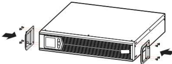
Рис 3.1 Установка угловых кронштейнов
