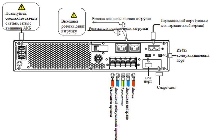
Рис 3. 3 Схема подключения для АБ-КР Л 11/6000+, АБ-КР 11/10000+
