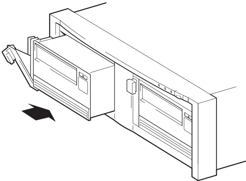
Рис. 4. Установка стримера
