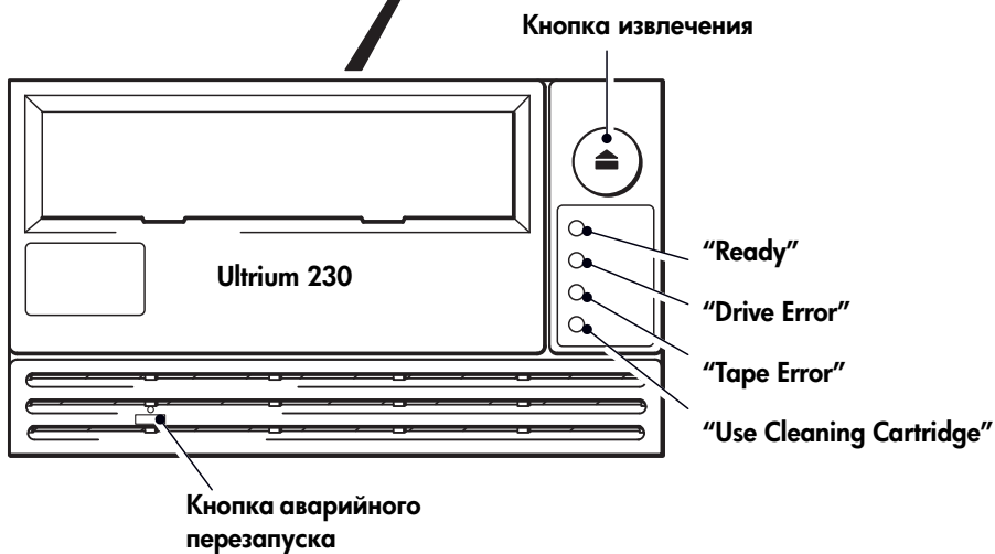
Рис. 7. Органы управления и индикаторы
