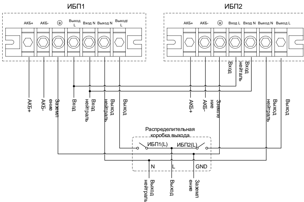
Рис 3.10 Схема подключения для ИБП 6 кВА/ 10 кВА при работе в параллель
