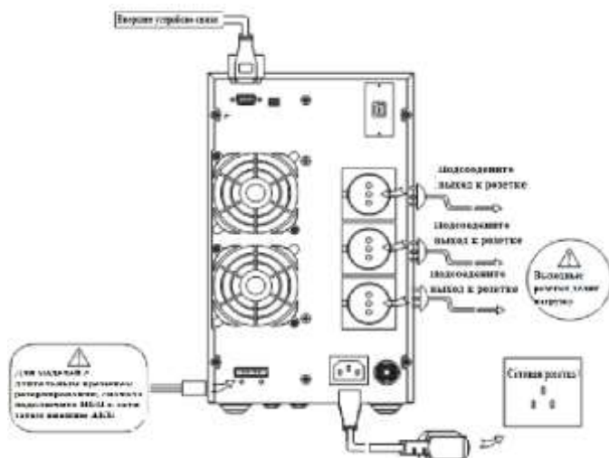
Рис 3.7 Схема подключения 2 кВА/ 3 кВА 2
