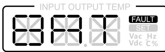
Рис 2.22 Ошибка АКБ
