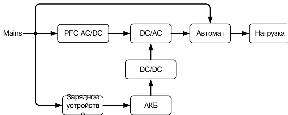
Рис 2.14 Принцип работы для (1-10 кВА)
