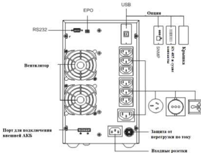
Рис 2.8 Задняя панель для ИБП 2 кВА/ 3 кВА
