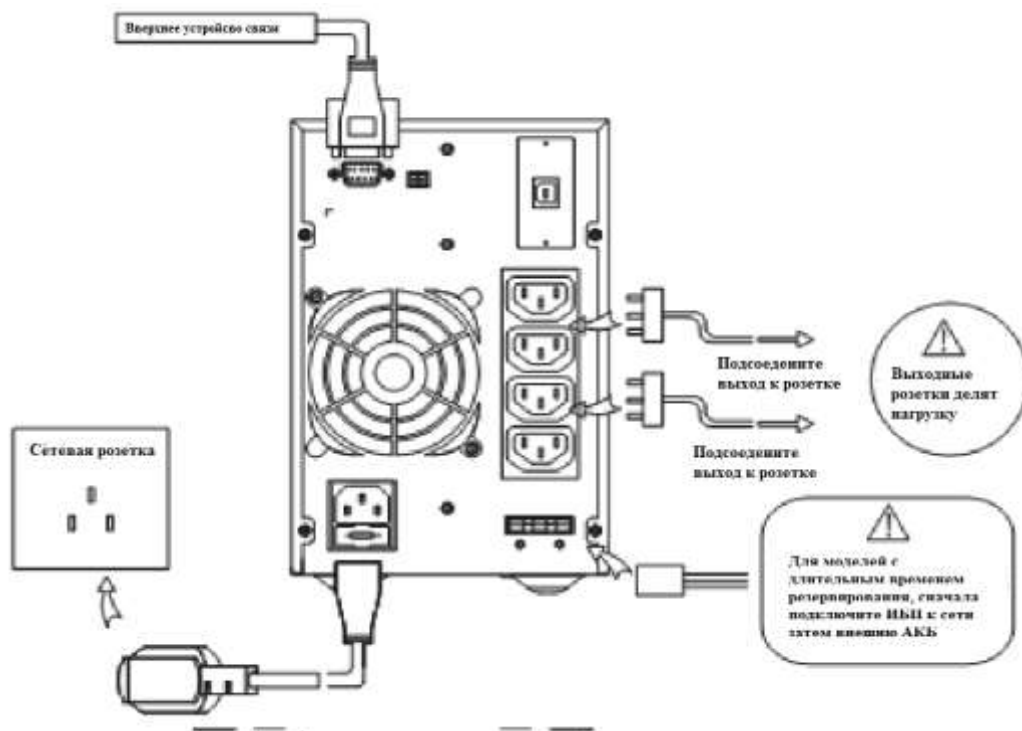
Рис 3.4 Схема подключения ИБП 1 кВА
