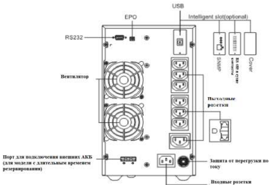
Рис 2.9 Задняя панель для ИБП 2.2 кВА/ 3 кВА
