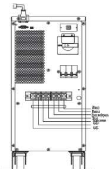
Рис 3.9 Схема подключения ИБП 6 кВА/ 10 кВА стандартная модель
