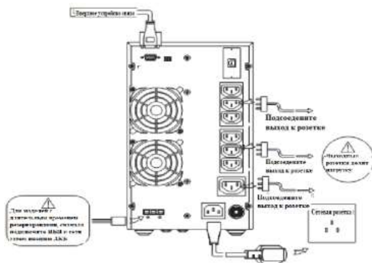
Рис 3.6 Схема подключения 2 кВА/ 3 кВА 1
