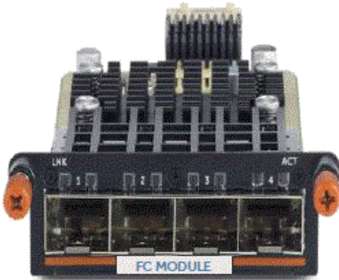
Figure 1-3. FC FlexIO Modules
